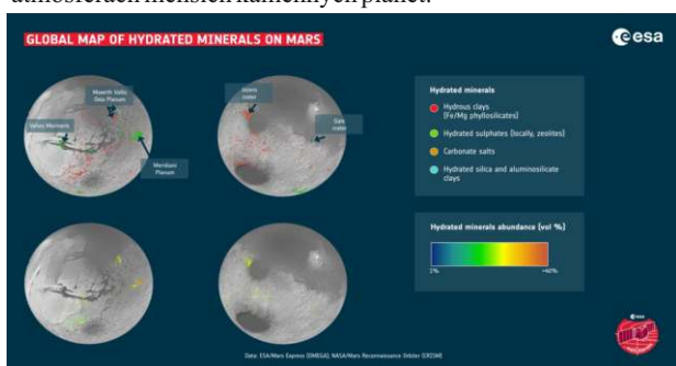
Mapa vodních minerálů na planetě Mars.
